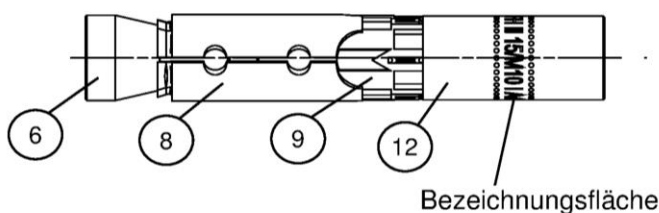
Innengewindeanker FH II 12 M6-I oder M8-I FH II 15 M10-I oder M12-I
