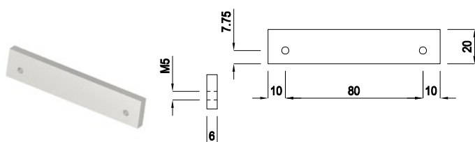
Stossverbinder aus Aluminium EN AW-6060 T66
