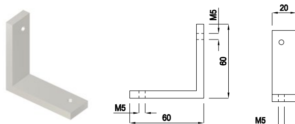
Eckverbinder aus Aluminium EN AW-6060 T66
